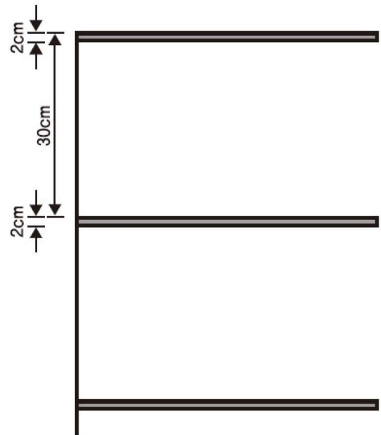
平面図
