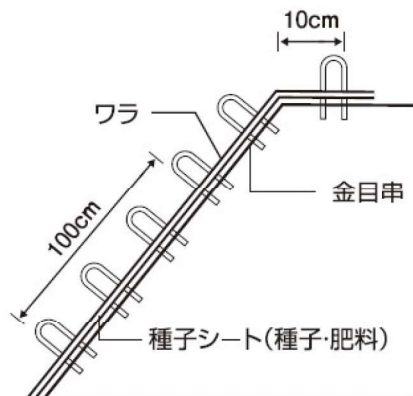
断面図
